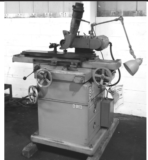
Hybco #1900 Tool Grinder
