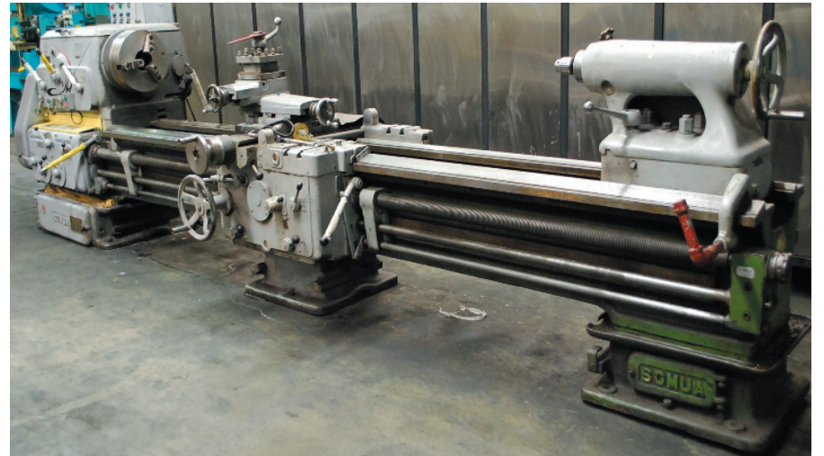
Somau (H.E.S.) 32" x 130" Lathe
